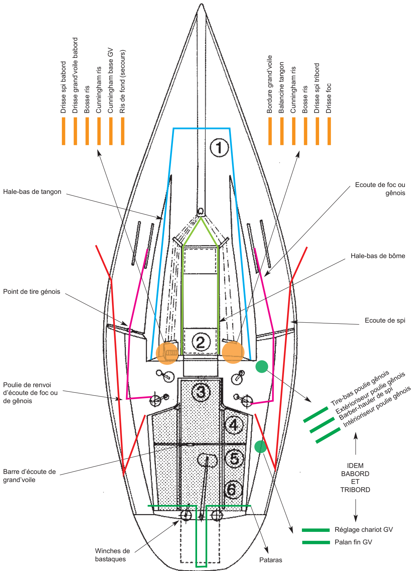
PLAN DE PONT DES PRINCIPAUX REGLAGES DU DB1 ATILLA - LA BOUÉE JAUNE
